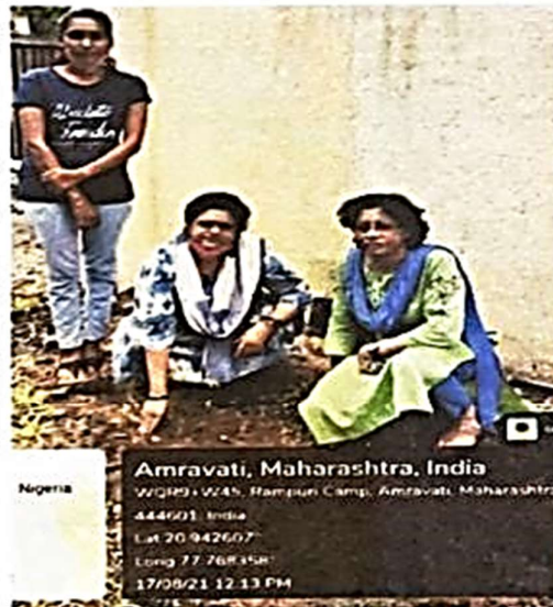
4)Neem
