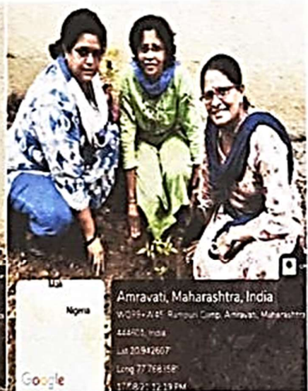
5)Neem
