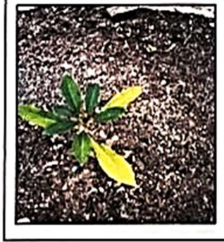
4) चाफा
